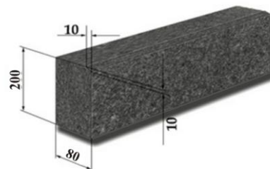
БОРДЮР ГП5 ТЕРМООБРАБОТАННЫЙ
